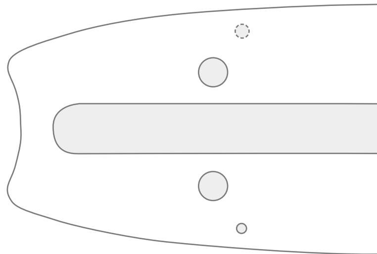
ANSCHLUSS: D025 Stihl 325" 1,3 mm und 1,6 mm 3/8" 1,6 mm
