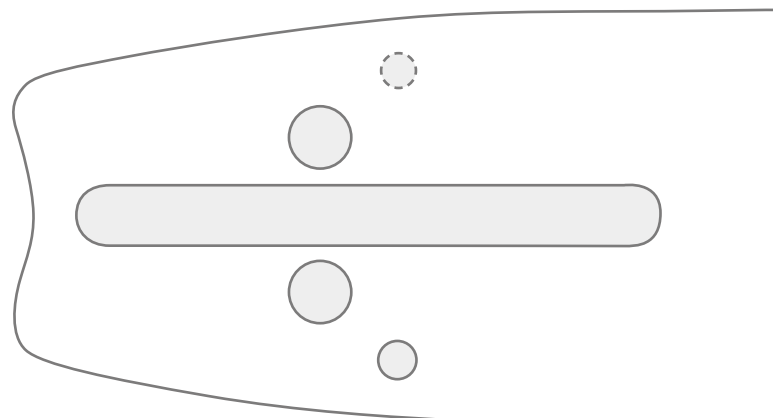
ANSCHLUSS: A095, K095 Dolmar, Husqvarna, Solo und andere 325" 1,3 mm und 1,5 mm 3/8" 1,5 mm
