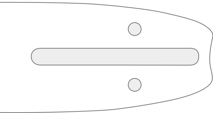
ANSCHLUSS: A041, Z041 Dolmar, Makita, Echo und andere 3/8" hobby 1,1 mm und 1,3 mm
